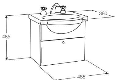
Conjunto lavatorio 48 cm y mueble de colgar
