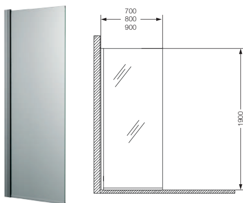
Mampara alta abatible. Vidrio transparente 8 mm. Perfil de aluminio brillante.
