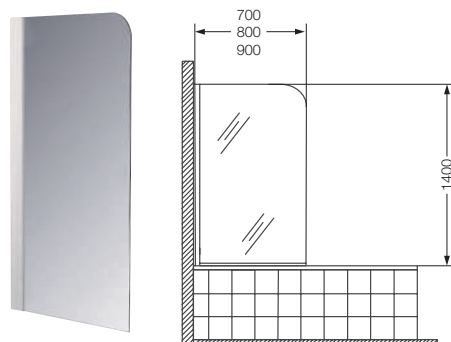
Mampara baja fija. Vidrio transparente 8 mm. Perfil aluminio brillante. Low folding screen. Grinding glass screen 8 mm. Bright aluminum perfil. NM7FA 01 (700 x 1400) NM8FA 01 (800 x 1400) NM9FA 01 (900 x 1400)
