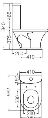
Depósito doble descarga - con válvula armada Double flush tank, with assembled valve DUWXF B / BE / S
