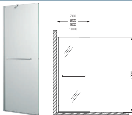
Mampara alta fija. Con toallero. Vidrio transparente 10 mm. Perfil de aluminio brillante.
