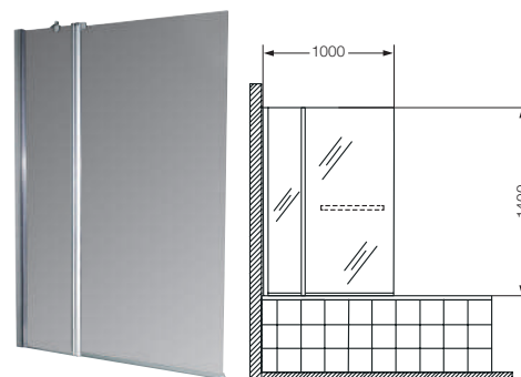
Mampara baja rebatible con hoja fija. Vidrio esmerilado 6 mm. Perfil aluminio brillante. Low folding screen. Grinding glass screen 6mm. Bright aluminum perfil. NM02Y 01 (1000 x 1400 mm)
