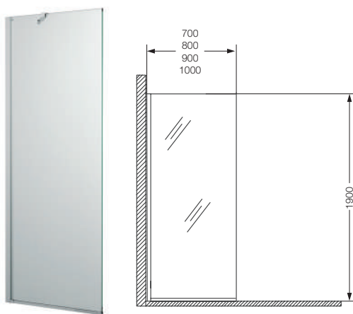
Mampara alta fija. Vidrio transparente 10 mm. Perfil de aluminio brillante.
